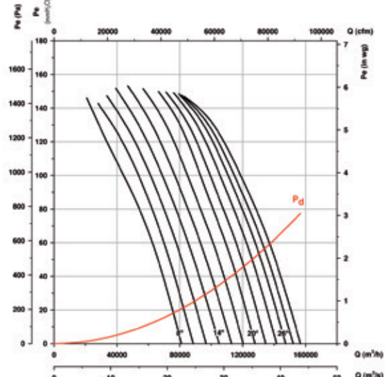
HTP-125-4T
