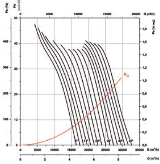
HTP-71-4T
