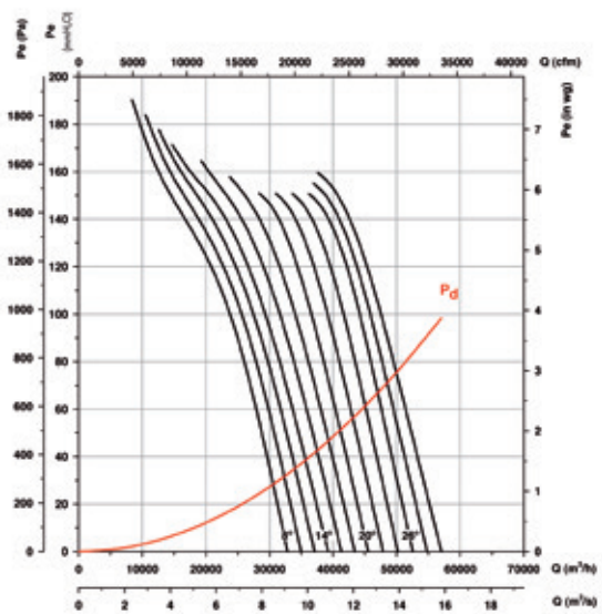
HTP-71-2T
